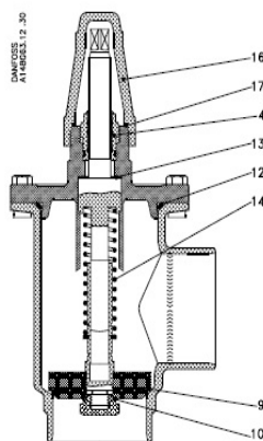
Fig. 1, SCH 50-100
