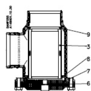
Fig. 1, STA 40-300
