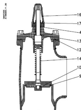
Fig. 2, SCH 125-200
