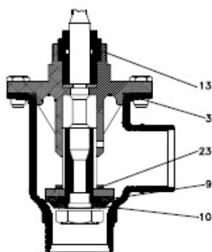
Fig. 1, SCV 25-200
